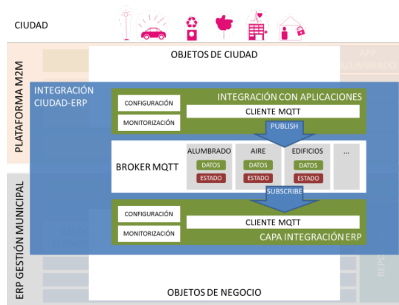
Ilustración 9. Ejemplo Vertical de Alumbrado en la Integración sistema M2M con el ERP
